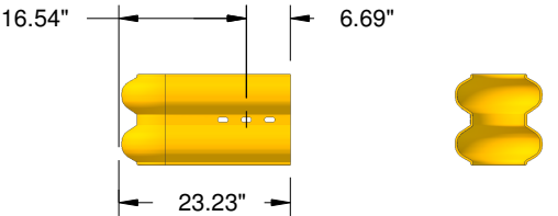
SSEE OPTIONAL END CAP
